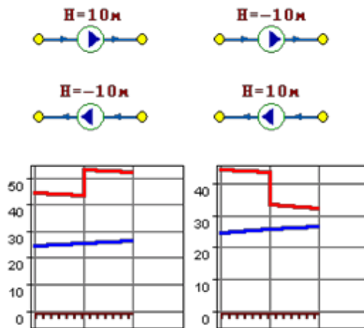
Рисунок 3.2.15. Пьезометрические графики
