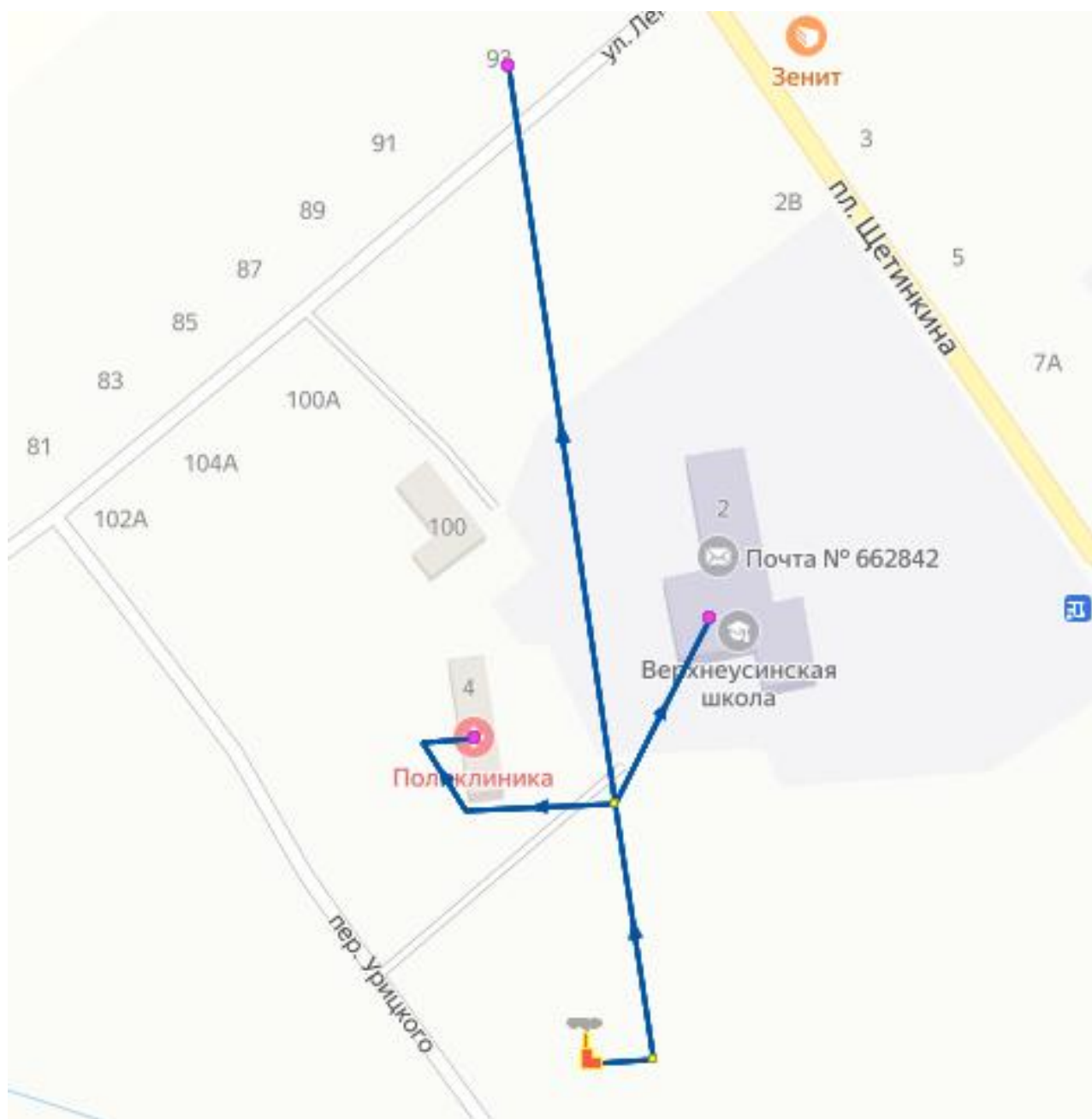
1.3.2.16 Схема тепловой сети от источника тепловой энергии Котельная с. Верхнеусинское
