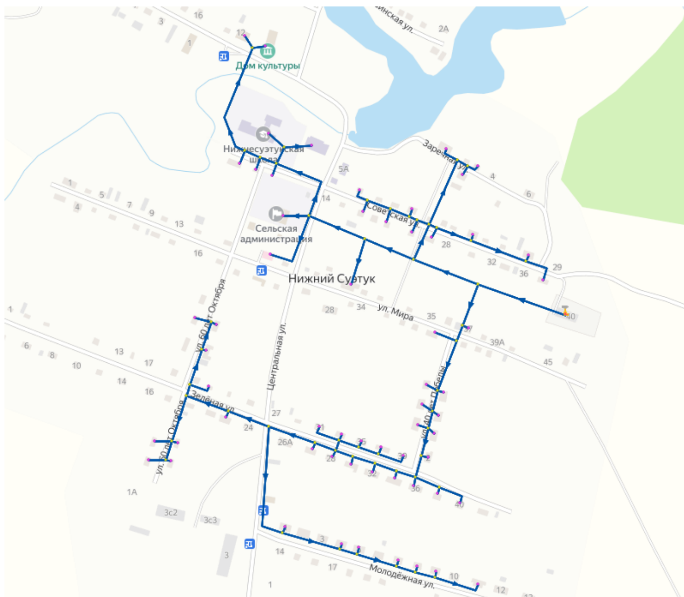
1.3.2.8 Схема тепловой сети от источника тепловой энергии Котельная с. Нижний Суэтук
