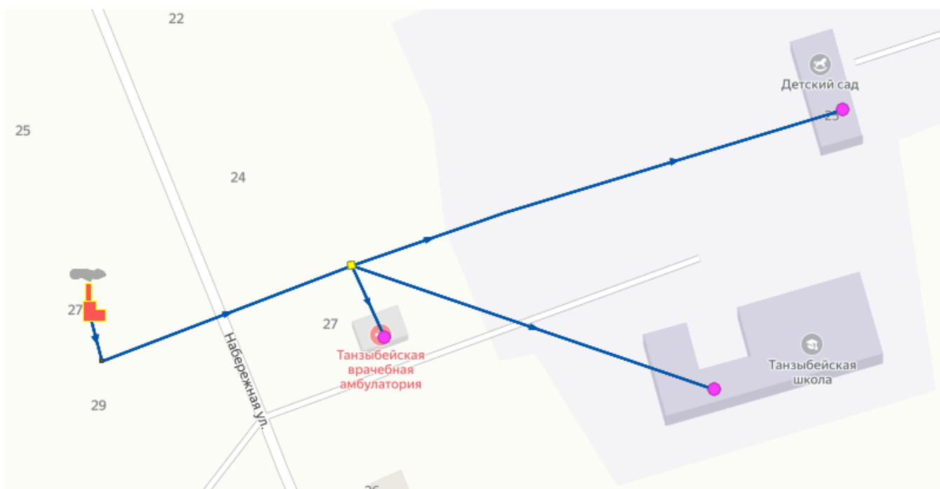
1.3.2.14 Схема тепловой сети от источника тепловой энергии Котельная п. Танзыбей
